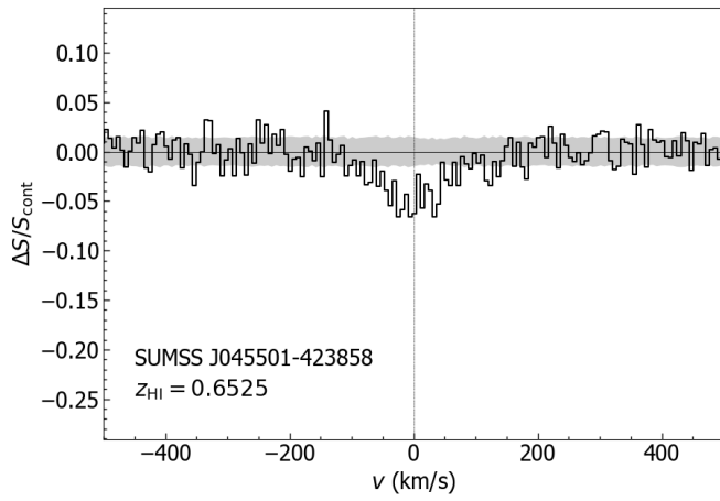
8. SUMSS J045501-423858
