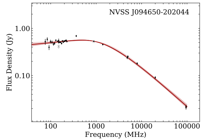
16. NVSS J094650-202044
