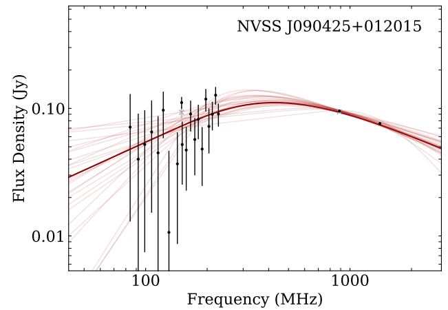
12. NVSS J090425+012015
