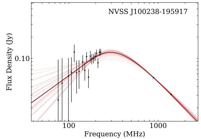
17. NVSS J100238-195917
