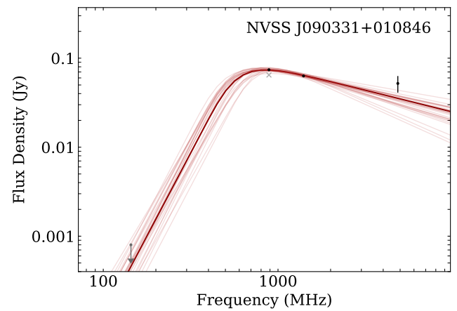
11. NVSS J090331+010846
