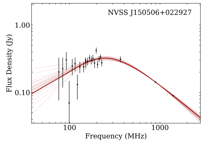
19. NVSS J150506+022927
