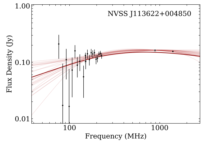
18. NVSS J113622+004850
