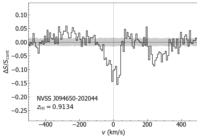
16. NVSS J094650-202044
