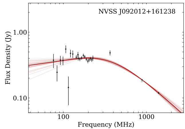
15. NVSS J092012+161238
