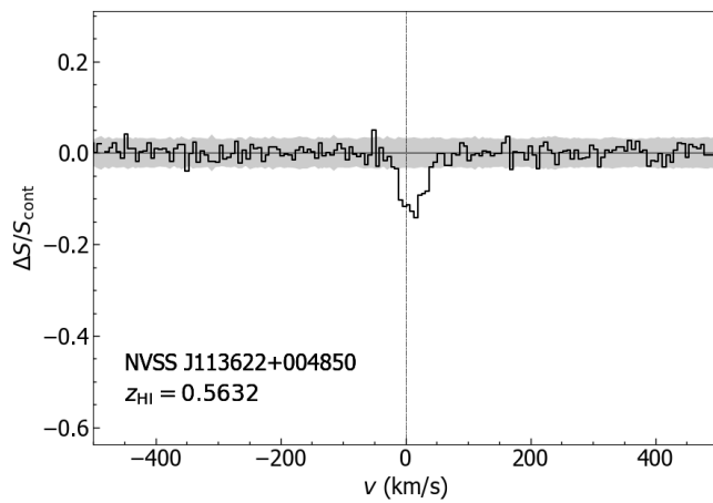
18. NVSS J113622+004850
