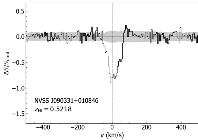
11. NVSS J090331+010846
