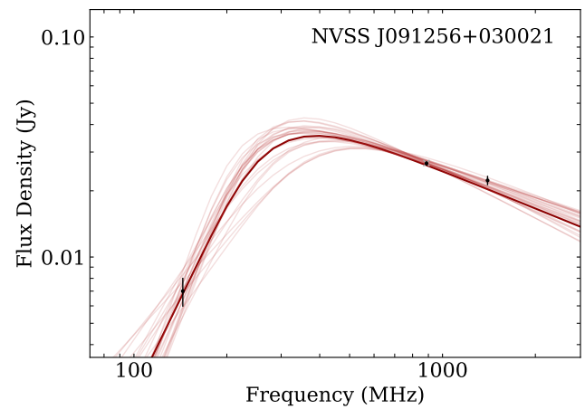
13. NVSS J091256+030021
