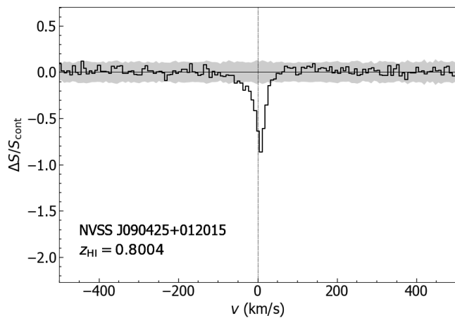
12. NVSS J090425+012015
