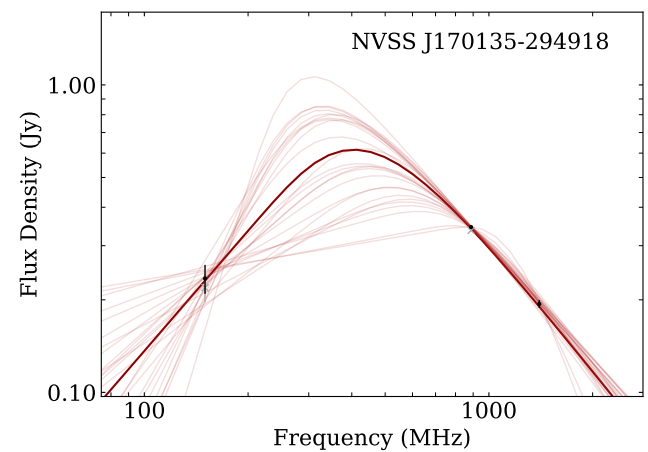
20. NVSS J170135-294918
