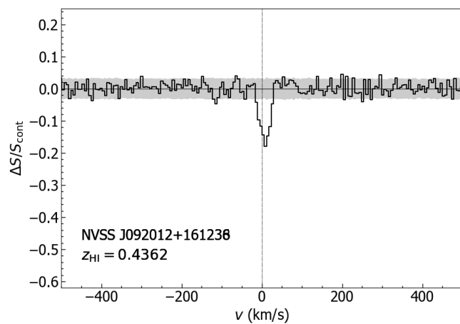
15. NVSS J092012+161238
