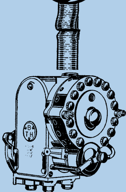
AV14 Magneto
